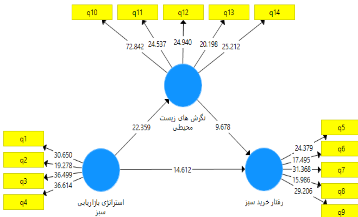
شکل ۲: معناداری مدل
