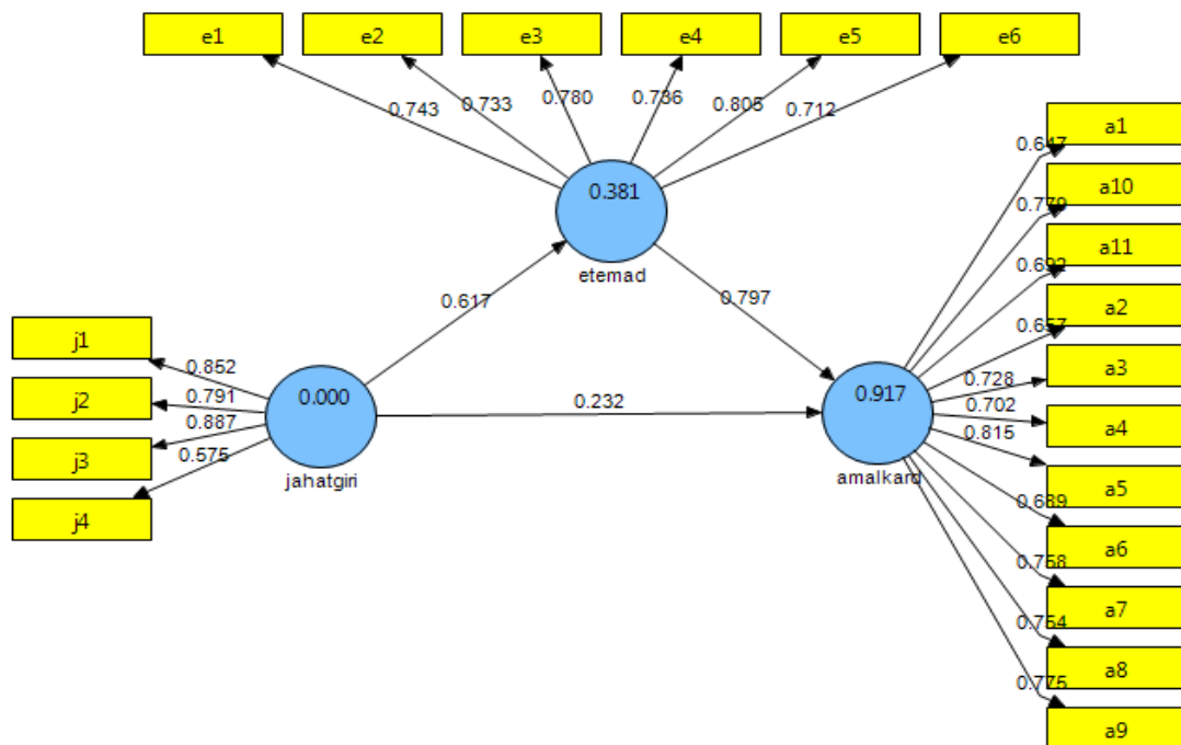
شکل ۲- ضرایب مسیر استاندارد مدل مفهومی پژوهش
