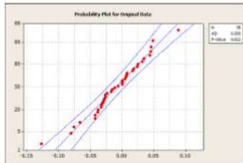
شکل ۱۰.۴: نمودار نرمالیتی باقیمانده های مدل رگرسیونی \Delta s_t^T = a s_{t-1}^T
