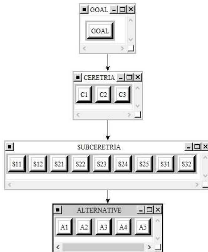
شکل ۱: نمودار AHP اولویت شاخص‌ها در نرم‌افزار سوپردسیژن
